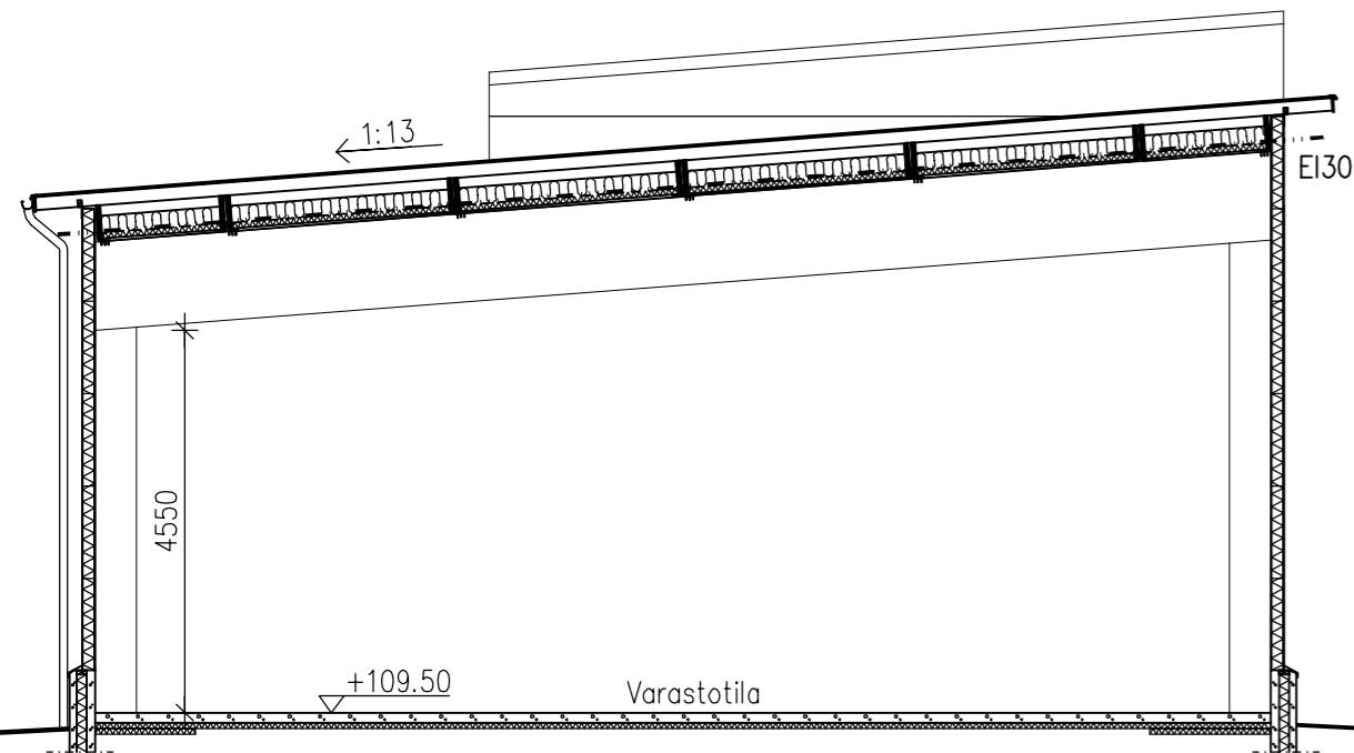
Leikkaus A-A
