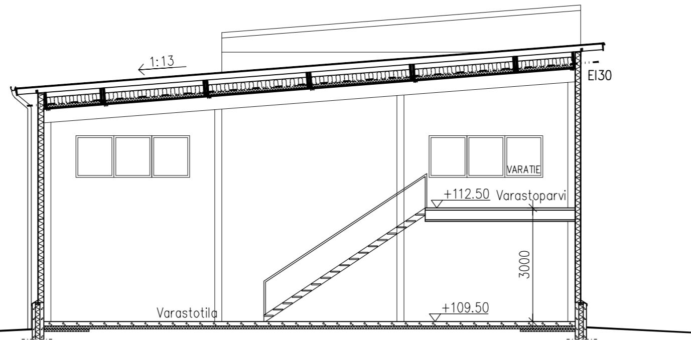
Leikkaus B-B
